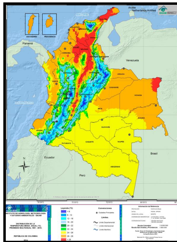
Mapa 2. Temperatura media del aire, media anual (1981-2010))
