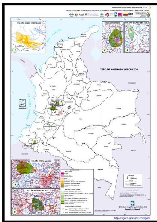
Mapa 7. Zonas de amenaza volcánica. Colombia
