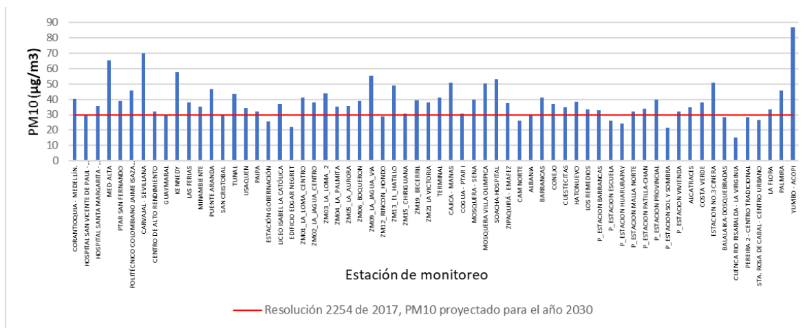
Gráfico 34. Promedio material particulado (PM10, \mu\text{g}/\text{m}^3 ) por estación de monitoreo, Colombia 2012 a 2019
